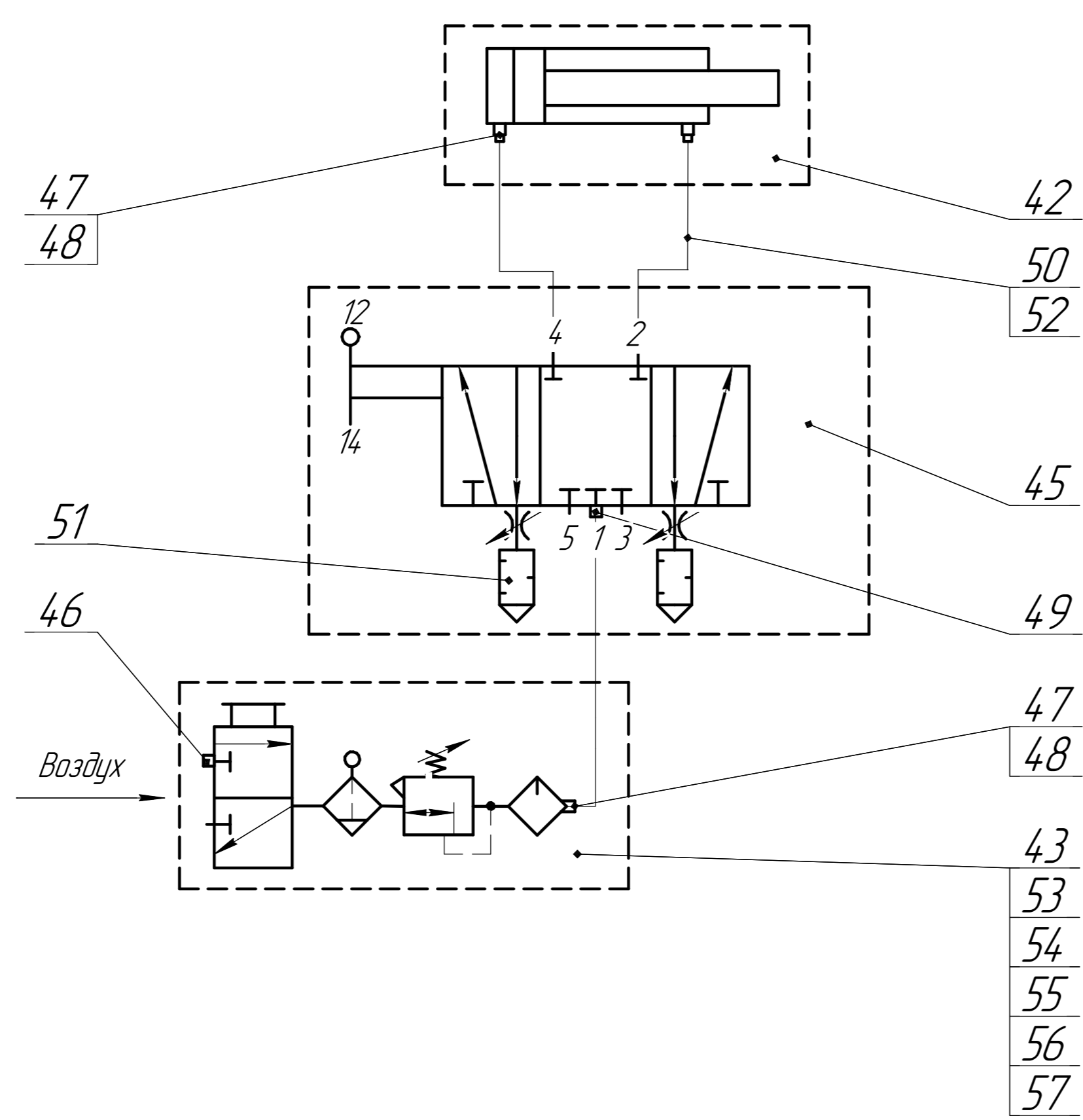
Схема пневматическая принцип.
